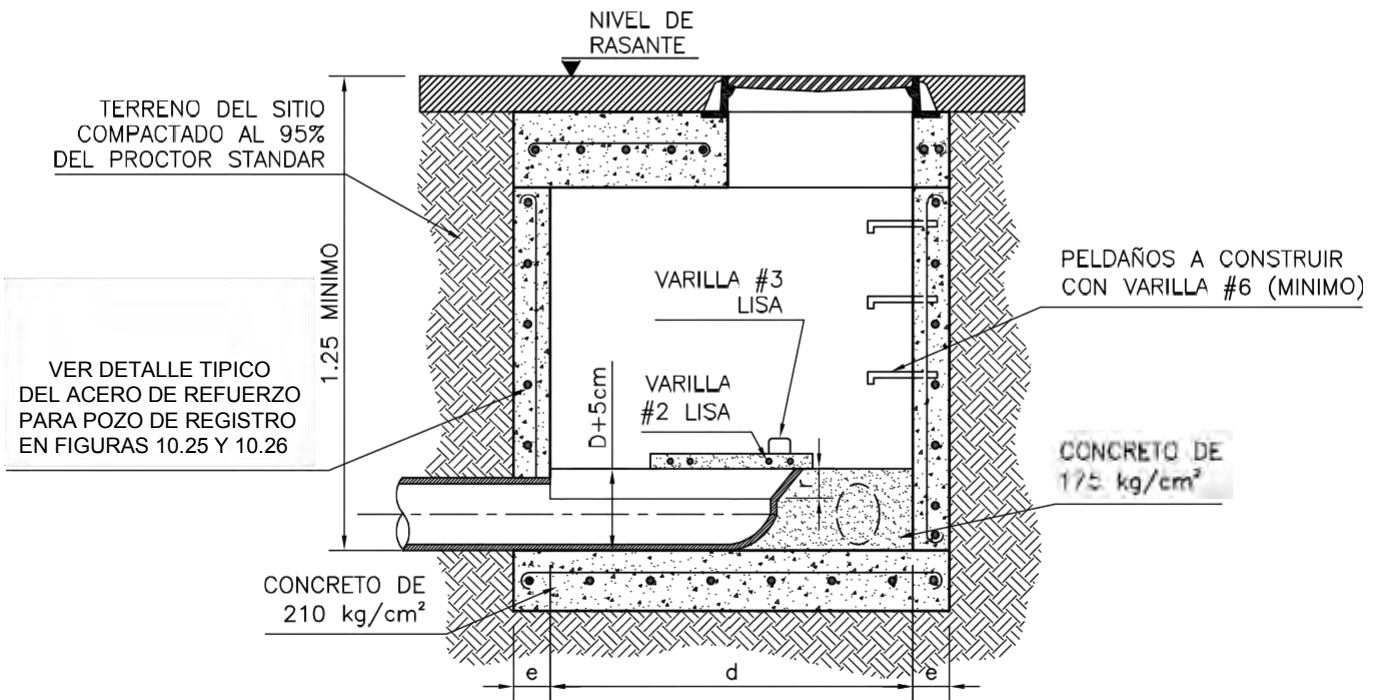
SECCION D-D
