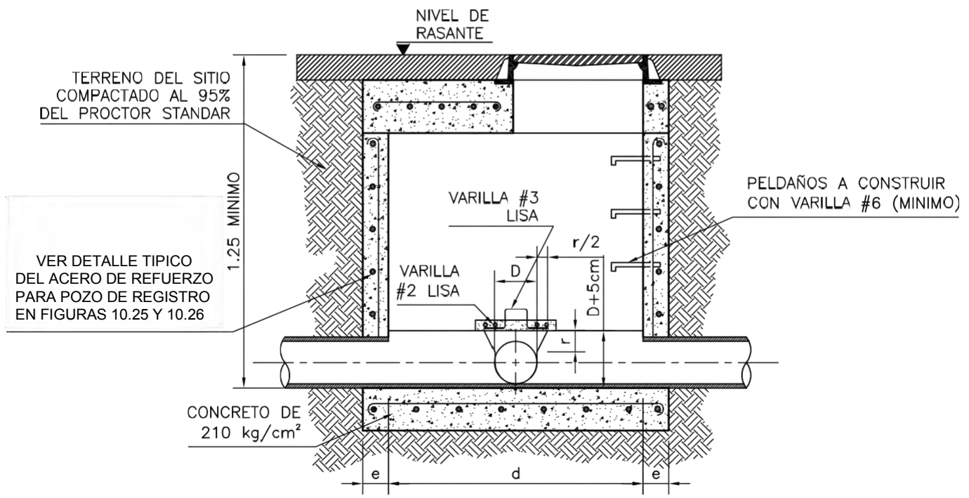
SECCION E-E
